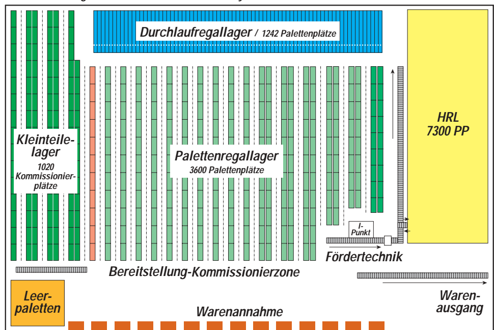
Layout: Kommissionierhalle
